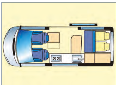
Grundriss merlin langer Radstand
